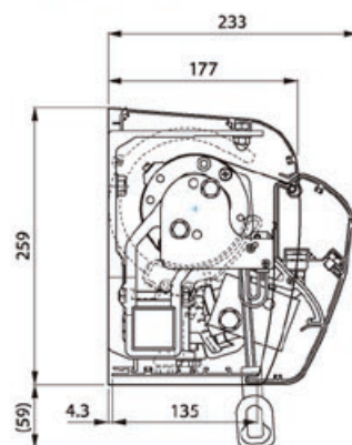
▼電手動タイプ
