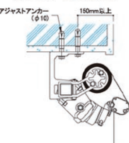
▼コンクリート造天井納まり
