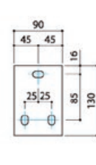
▼コンクリート造の場合
