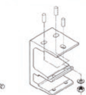
▼コンクリート天井納まり
